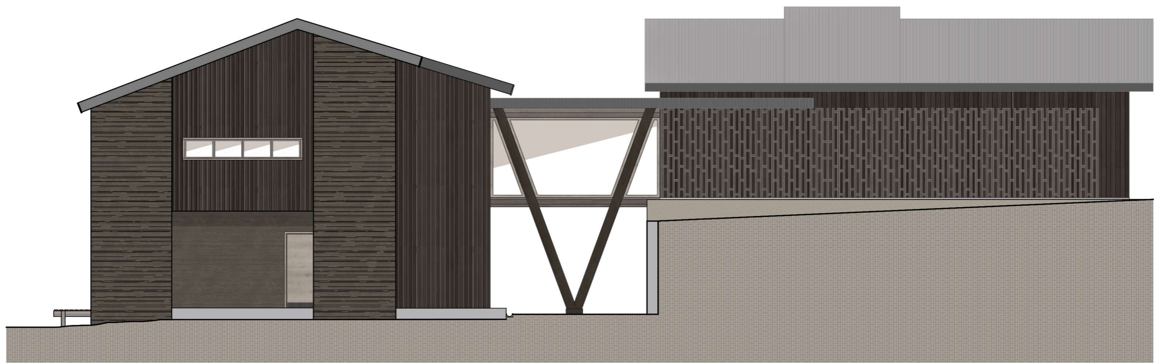
ELEVACIÓN SUR
