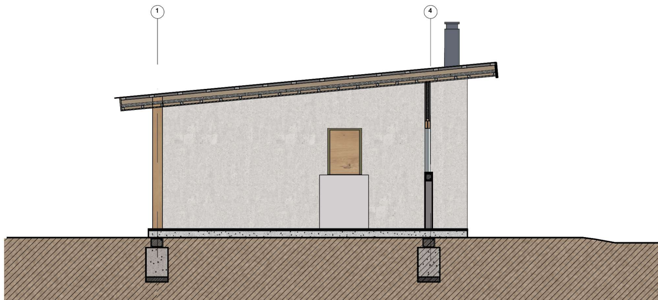
CORTE C-C' QUINCHO LP
