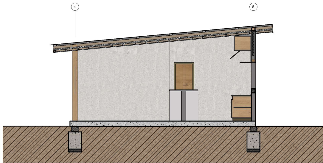
CORTE B-B' QUINCHO LP
