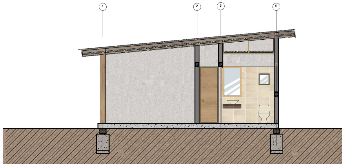
CORTE A-A' QUINCHO LP
