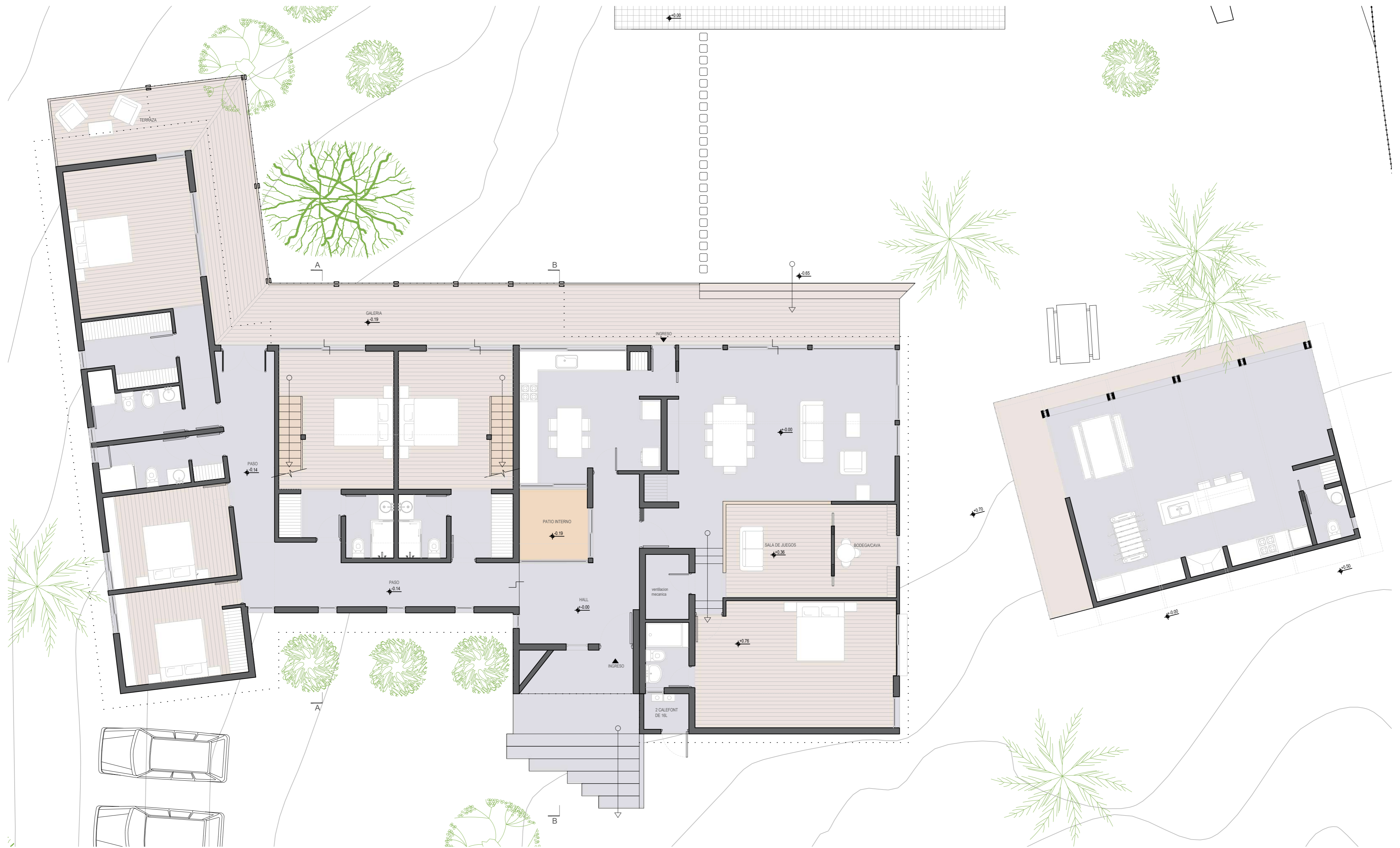
PLANTA BAJA CASA LP
