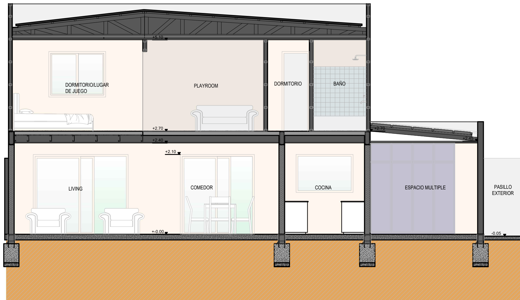
CORTE B-B CASA ALTO LOS CIPRESES
