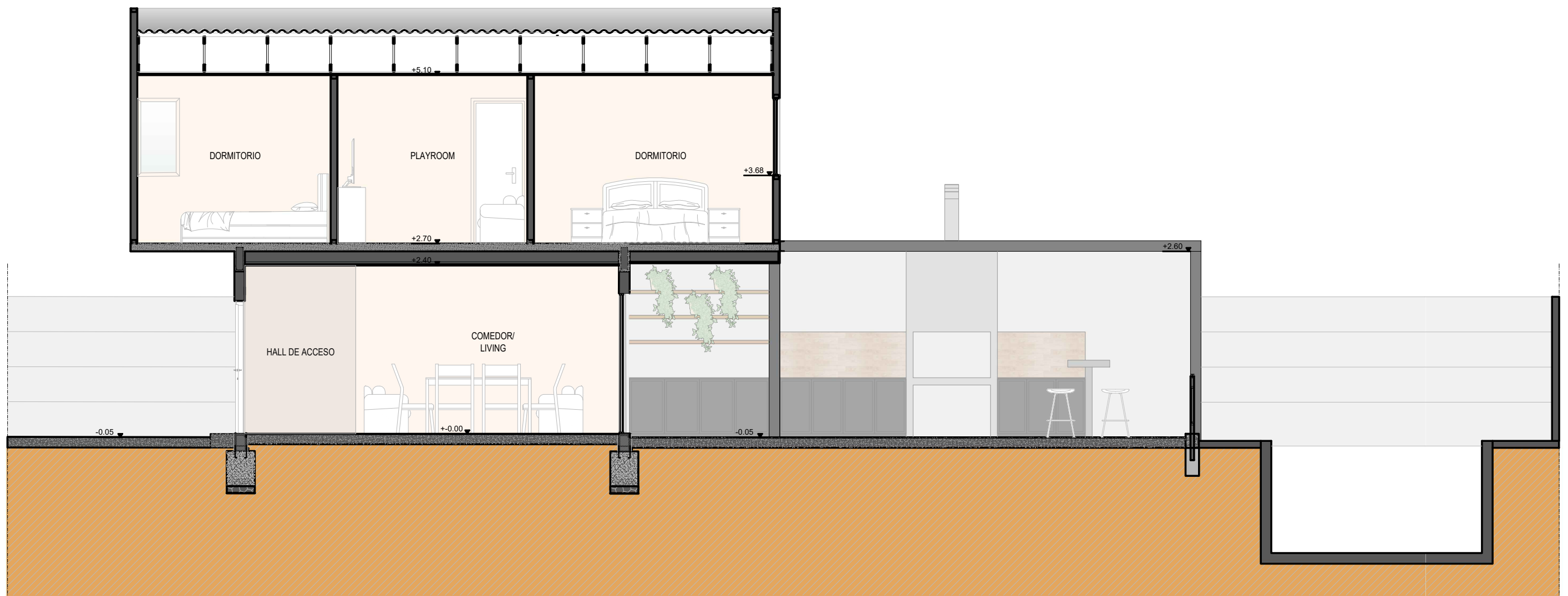
CORTE A-A CASA ALTO LOS CIPRESES
