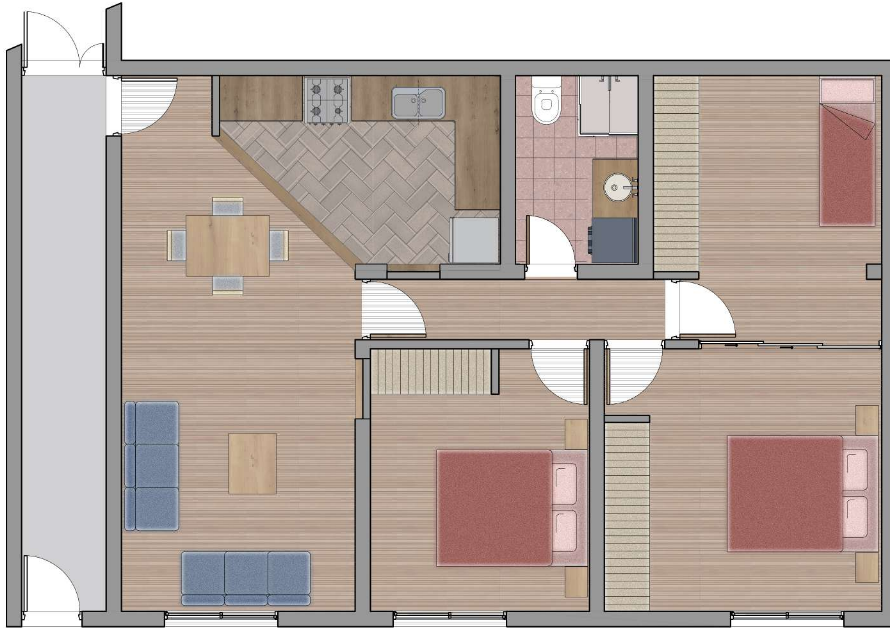
PLANTA ARQUITECTÓNICA CASA CALETA ABARBARCA
