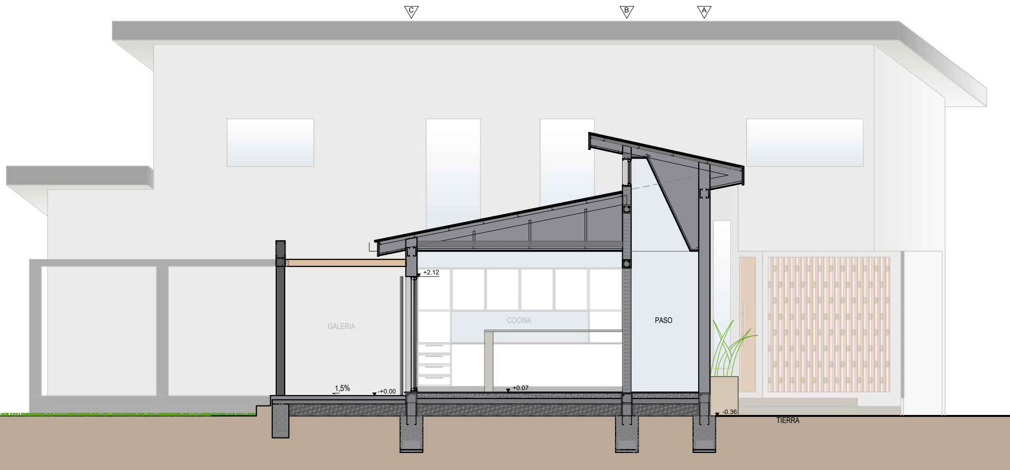
CORTE A-A CASA FL
